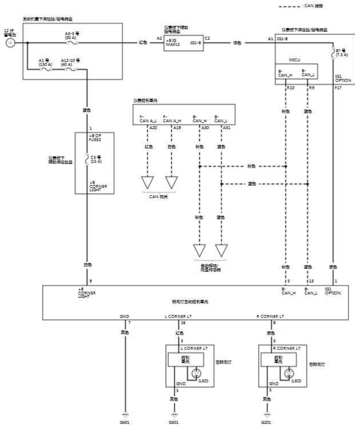
主动转向灯电路图
